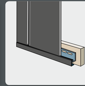
Ontwateringsprofiel
