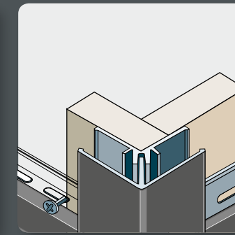
Buitenhoekprofiel
